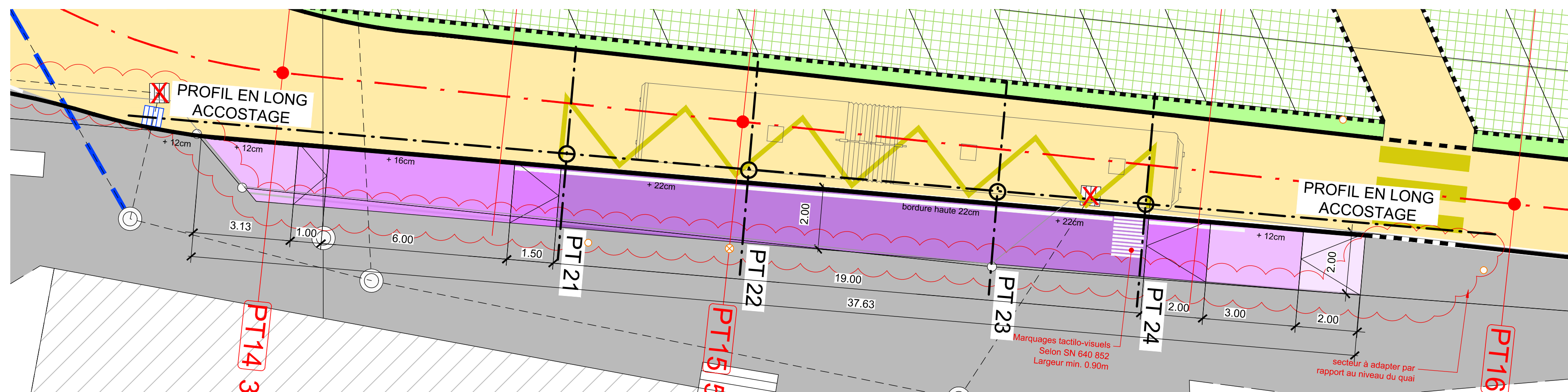
SITUATION - Arrêt de bus Ech. : 1:100
